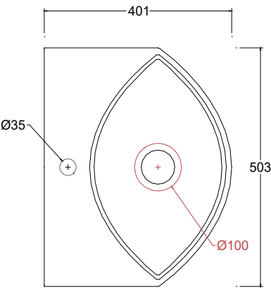
Vista superiore Baview
