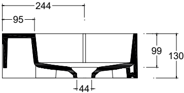
Sezione A-A Section A-A
